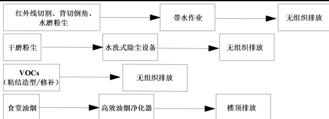
图 3-2 废气处理示意图
