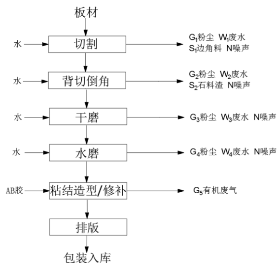
图 2-2 运营期工艺流程及产污节点图
