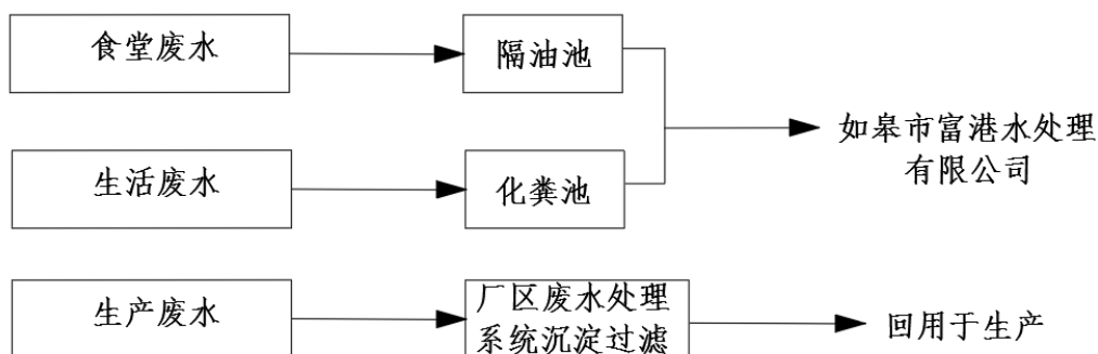
图 3-1 废水处理工艺流程图
