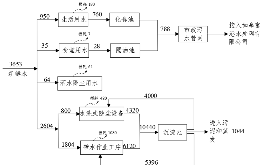
图 2-1 项目实际水平衡图
