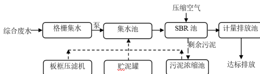
图 4-2 如皋市吴窑镇污水处理厂处理工艺流程图
