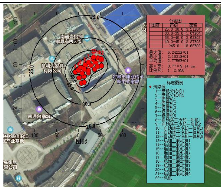
图 4-3 本项目等声级线图
