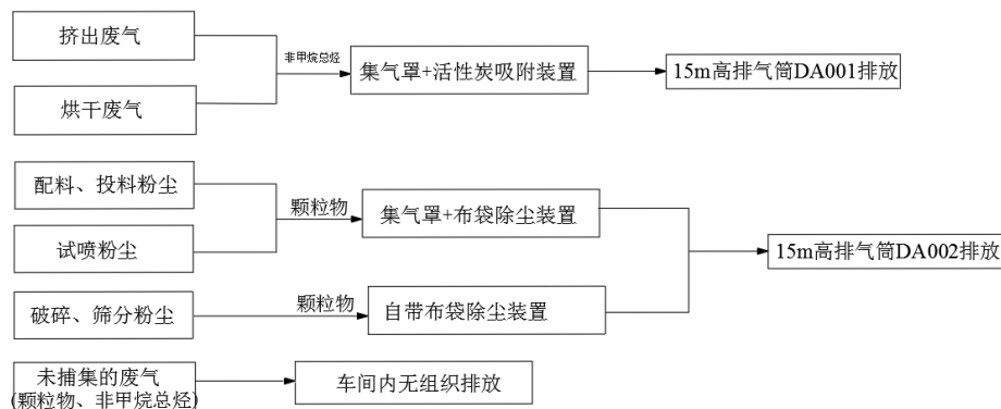
图 4-2 本项目废气处理工艺流程
