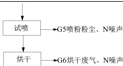
图 2-2-2 塑粉试喷过程工艺流程图
