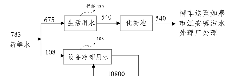
图 2-1 本项目水平衡图 (t/a)
