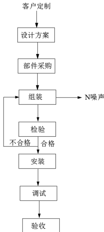
图 2-3 智能喷涂机组装生产工艺流程图
