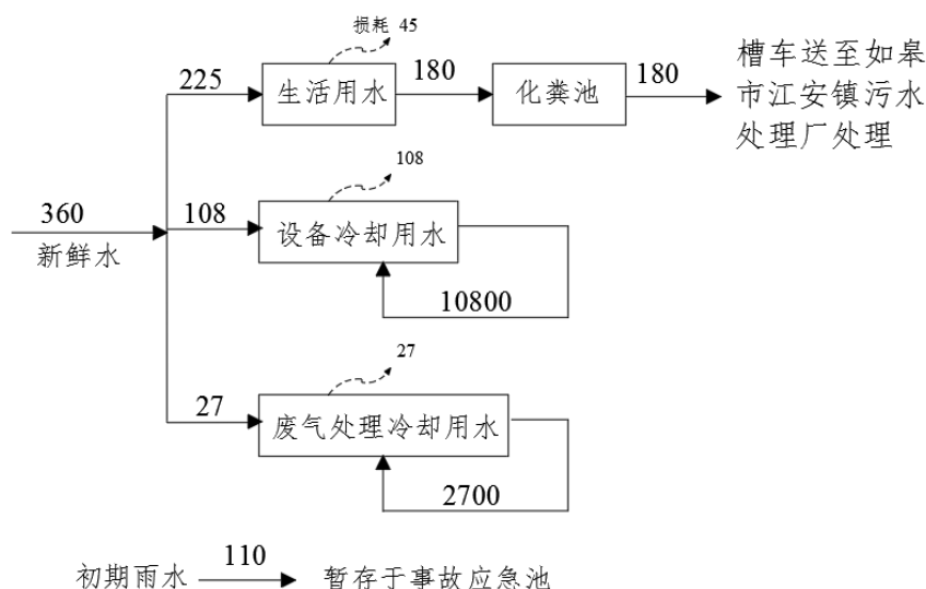
图 2-1 本项目水平衡图 (t/a)
