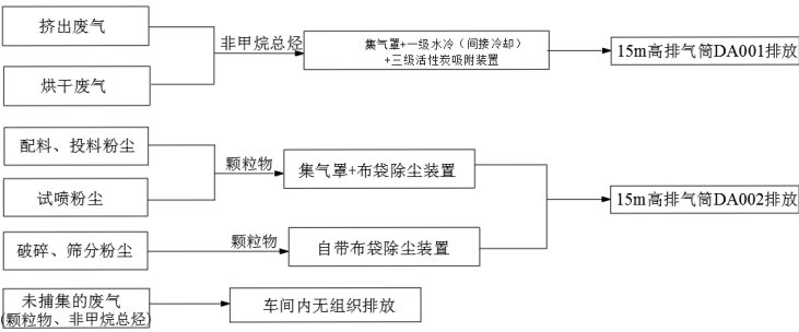
图 4-2 本项目废气处理工艺流程
