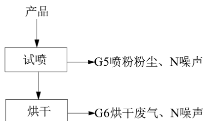
图 2-2-2 塑粉试喷过程工艺流程图
