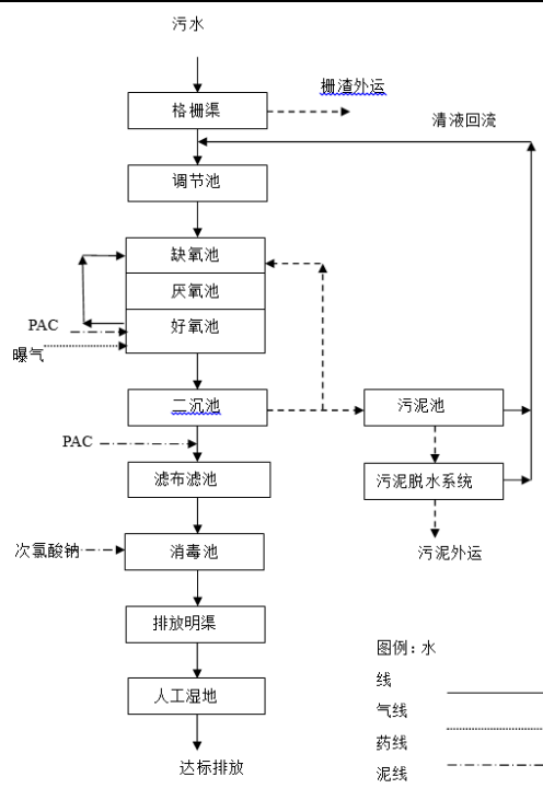
图 4-3 如皋市江安镇污水处理厂污水厂工艺流程图
