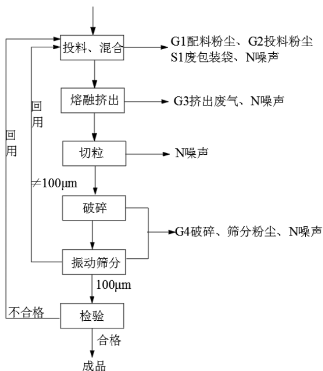
图 2-2-1 喷涂塑粉生产工艺流程图
