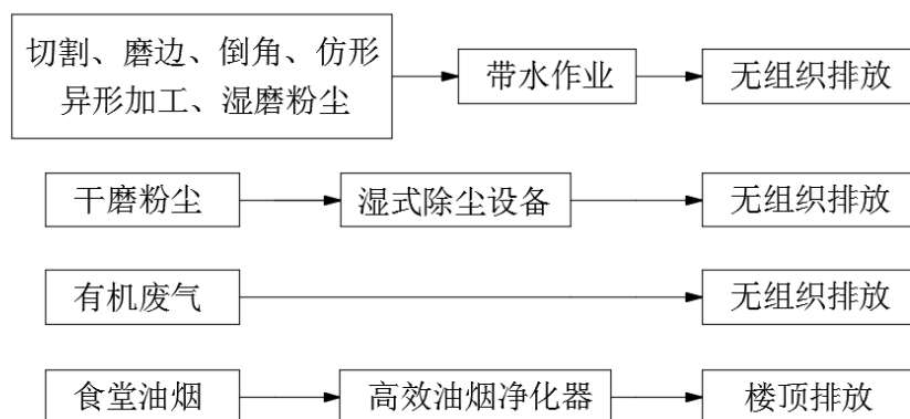
图 3-3 废气处理示意图
