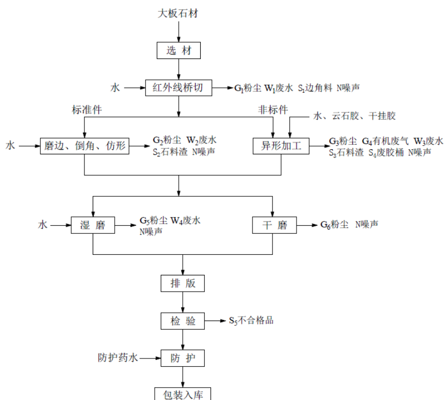
图 2-2 运营期工艺流程及产污节点图
