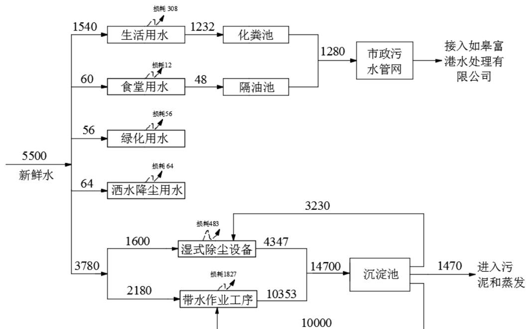
图 2-1 项目实际水平衡图
