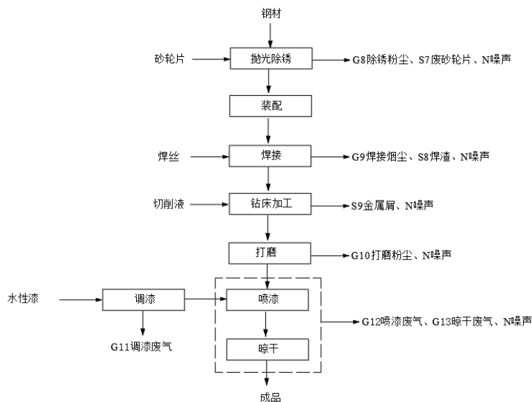
图 2-4 附件生产工艺流程图
