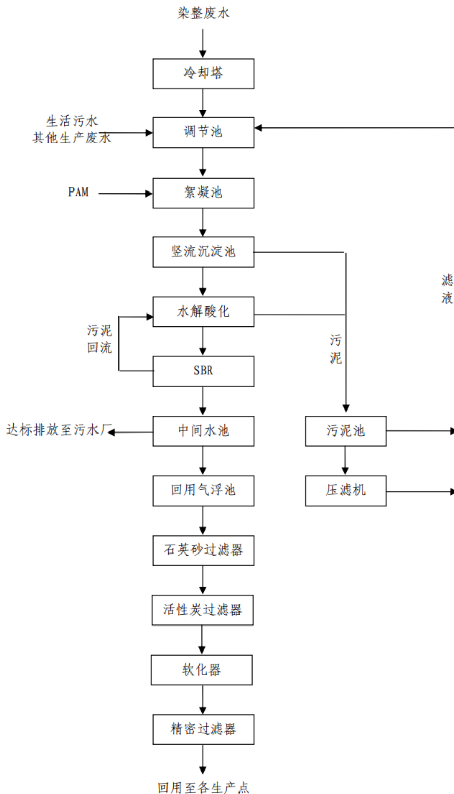
图 2-2 综合污水处理站工艺流程图
