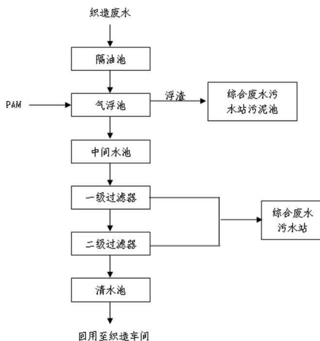
图 2-1 织造废水回用工艺流程图
